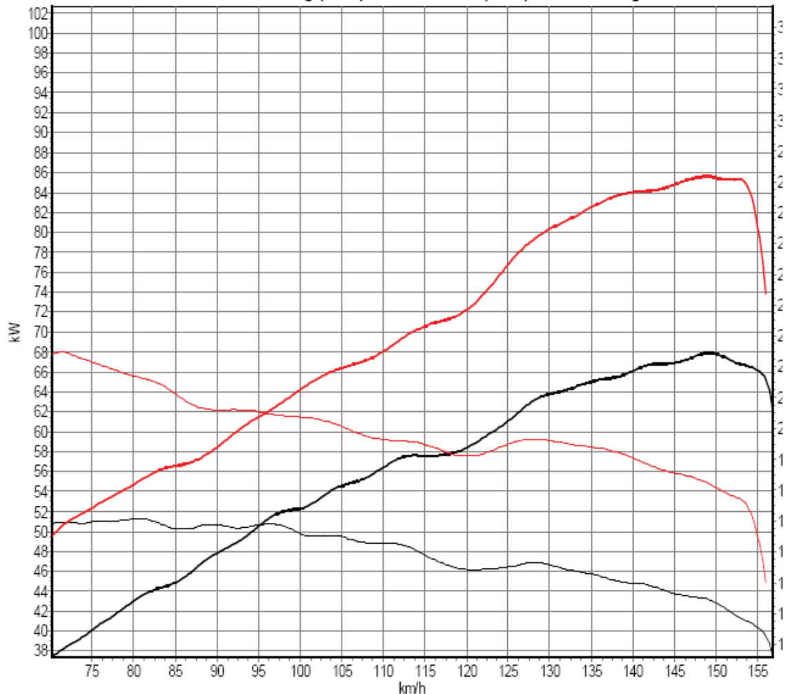
P-max Motorleistung (korr.) / Drehmoment (korr.) / Geschwindigkeit
